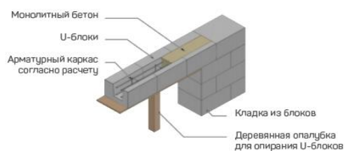
Схема изготовления перемычки из U-блоков «ЭКО»
